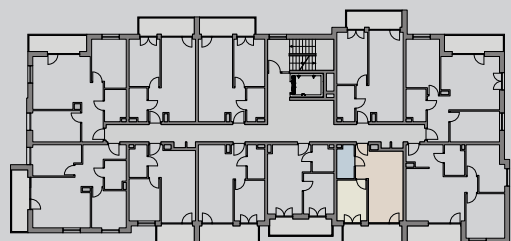
RZUT KONDYGNACJI
